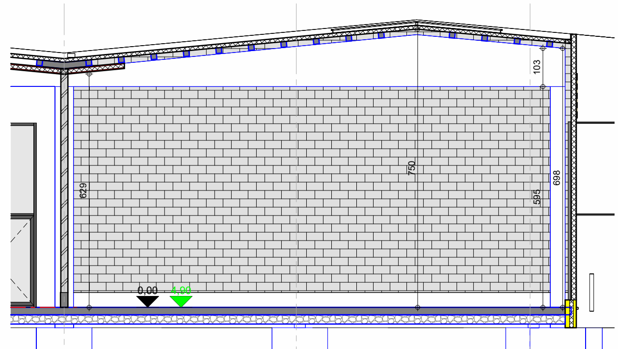
Doorsnede Unit A.8
