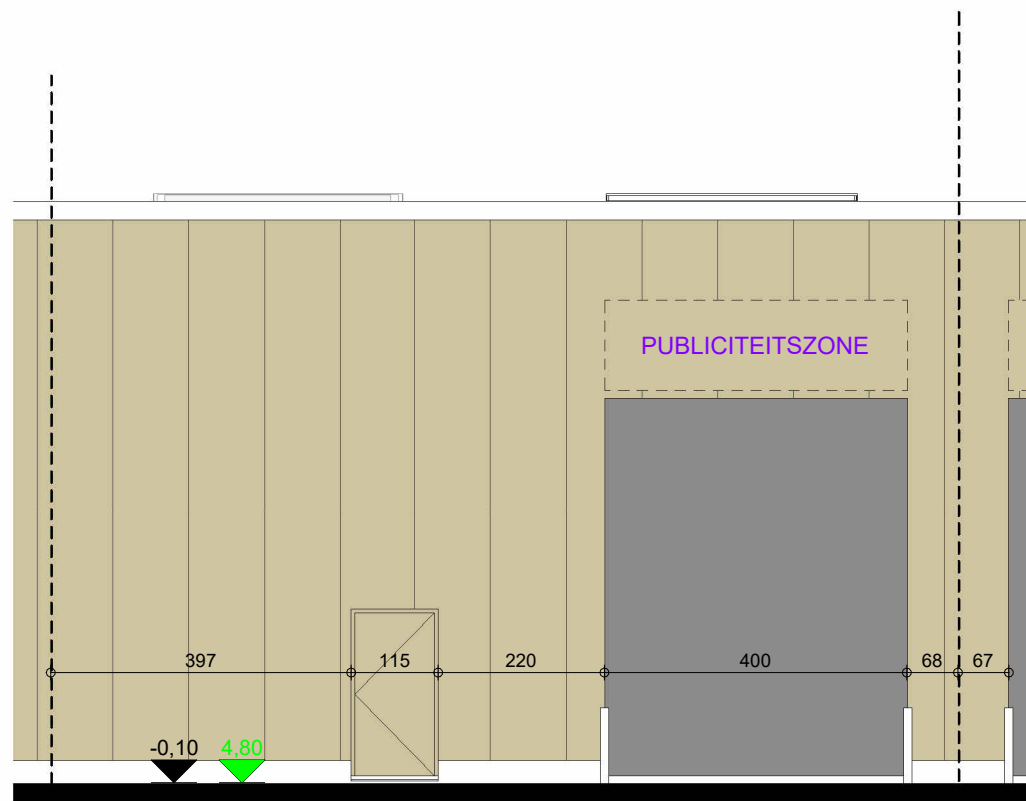
Oost gevel Unit A.8
