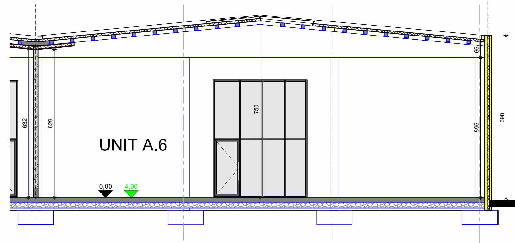
DOORSNEDE HA
